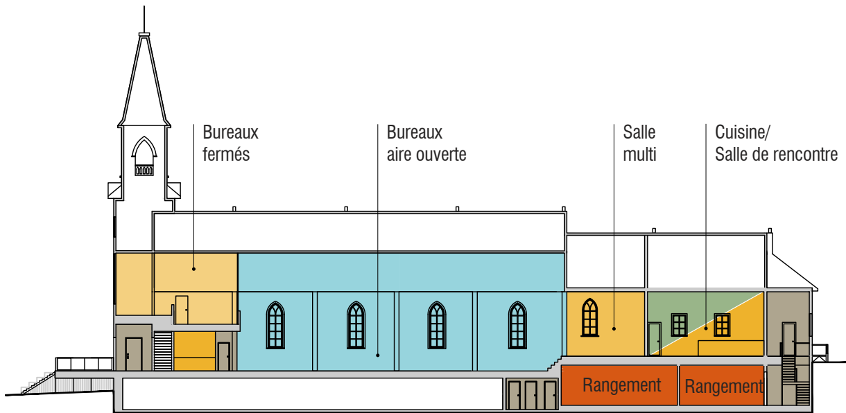
COUPE LONGITUDINALE
